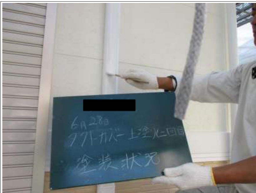
ダクトカバー 上塗り施工中(2回目)
