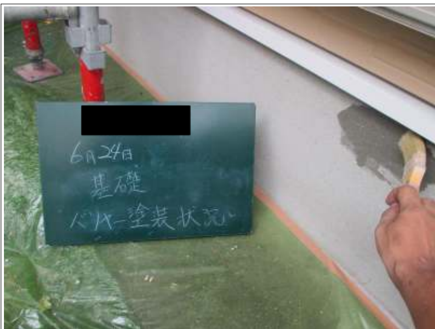
基礎 バリヤー施工中
