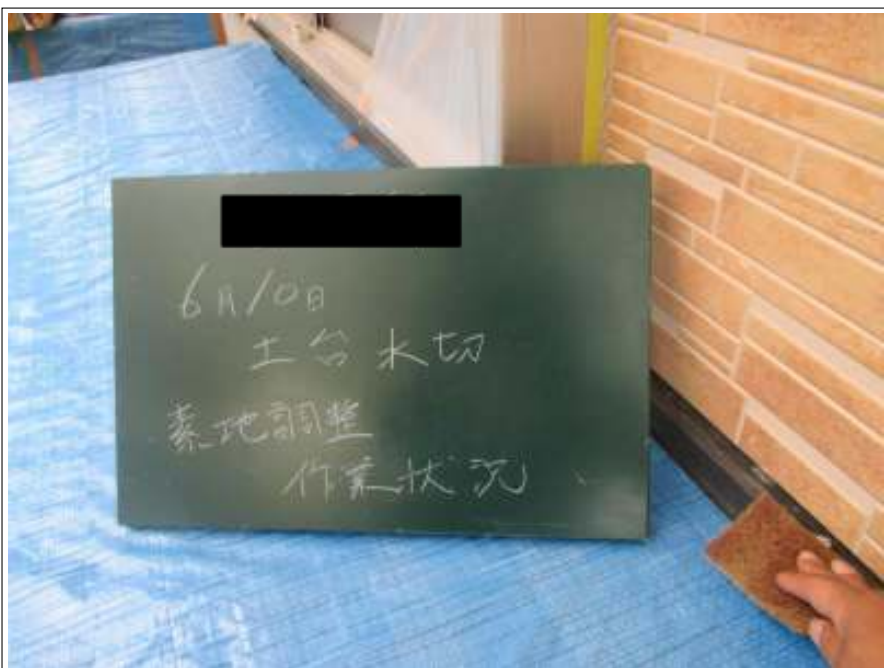
土台水切り 研磨紙ずり施工中
