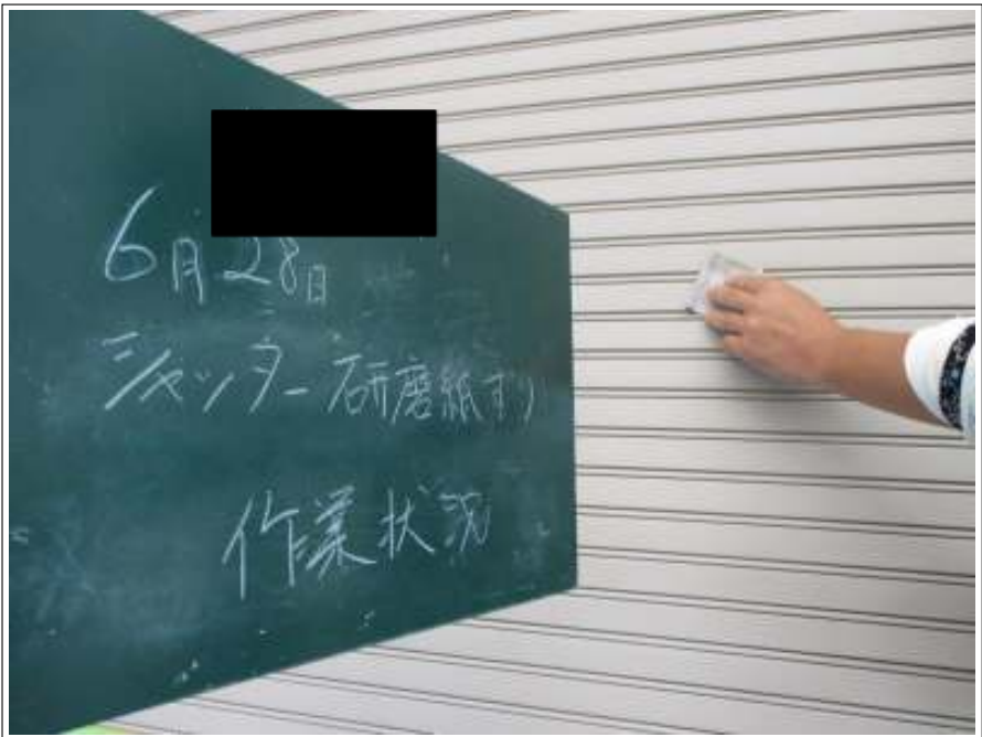
シャッター 研磨紙ずり施工中
